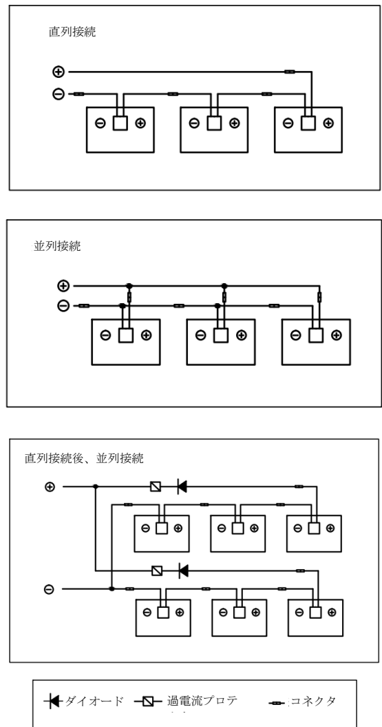
図 11 電氣的接続のイメージ図
