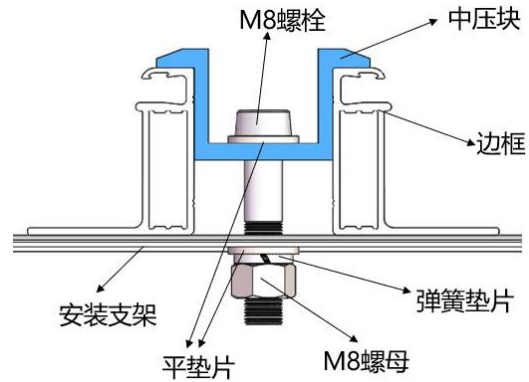
図10 中間クランプの取付イメージ図
