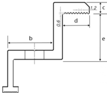
図8 エッジクランプの断面イメージ図
