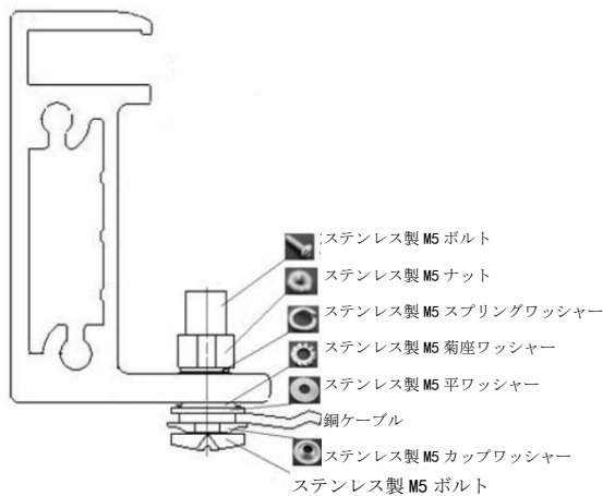
図 12 銅ケーブルによるアルミフレームの接地
