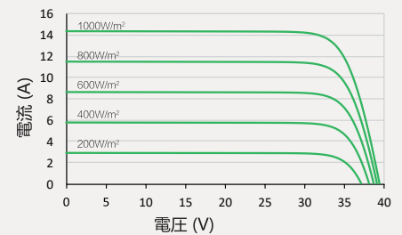
P-V 曲線 (450 W)
