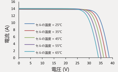
I-V 曲線 (430 W)
